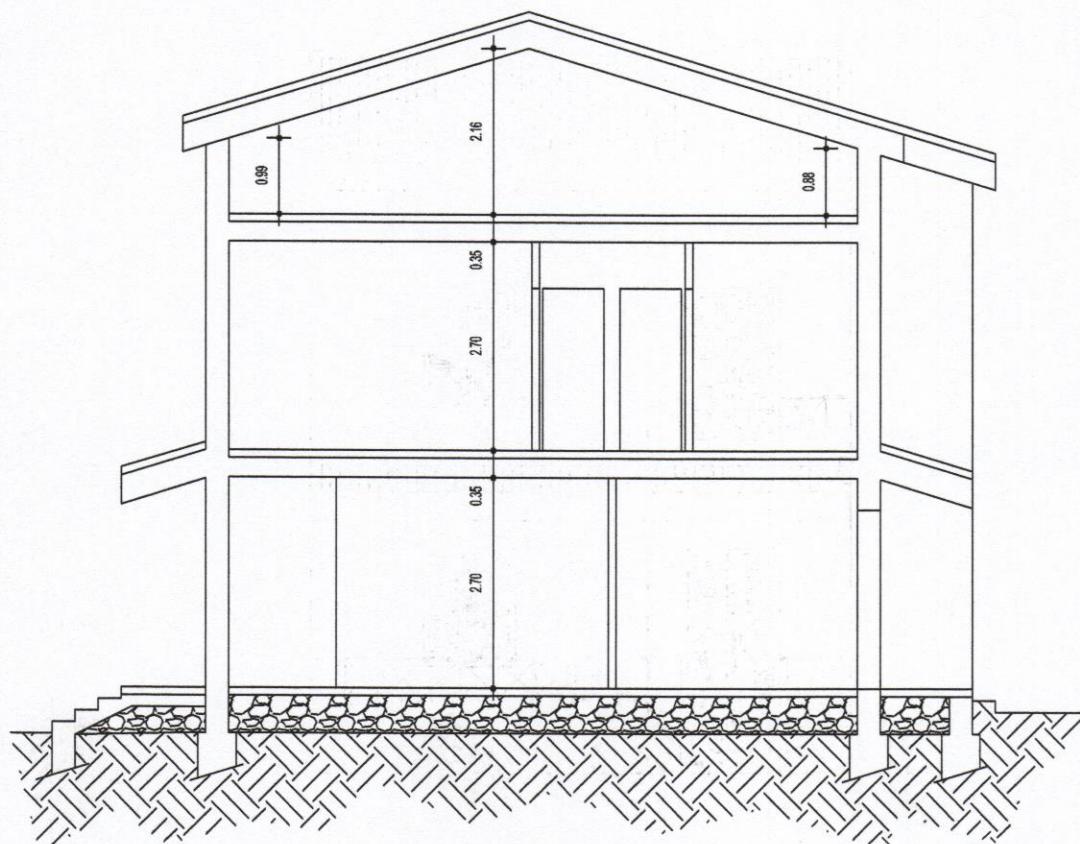
SEZIONE A-A
